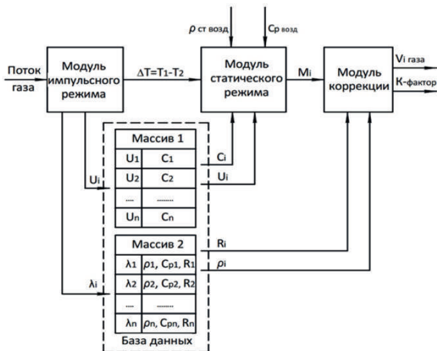
Рис.3. Структурная схема алгоритма работы датчика
